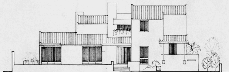
ALÇADO SUL
