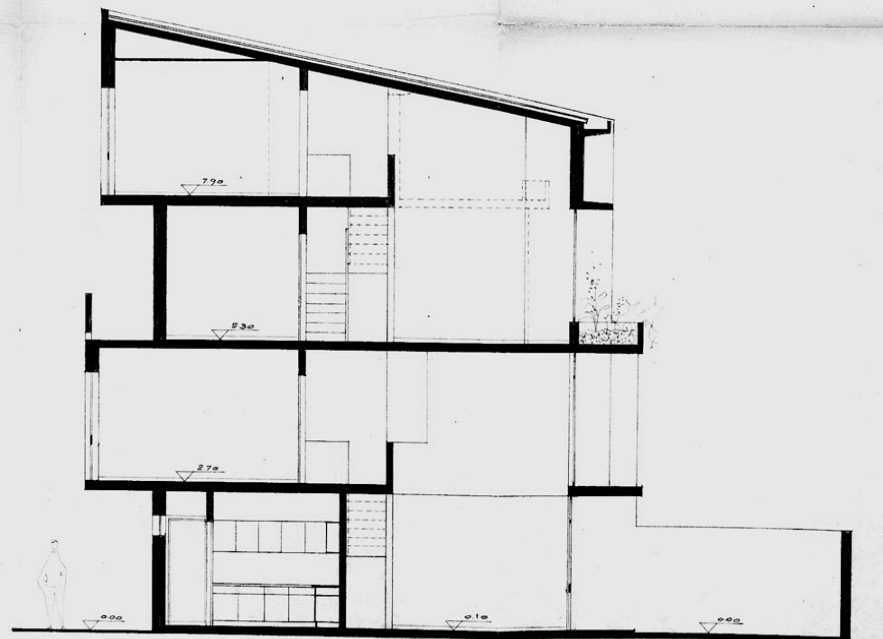
CORTE A-B
