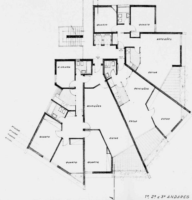
1º, 2º e 3º ANDARES
