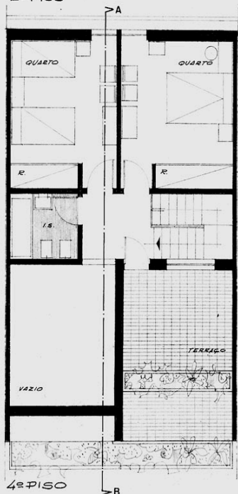
4º PISO
