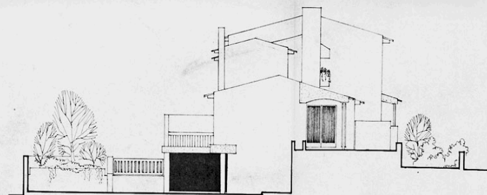
ALÇADO POENTE
