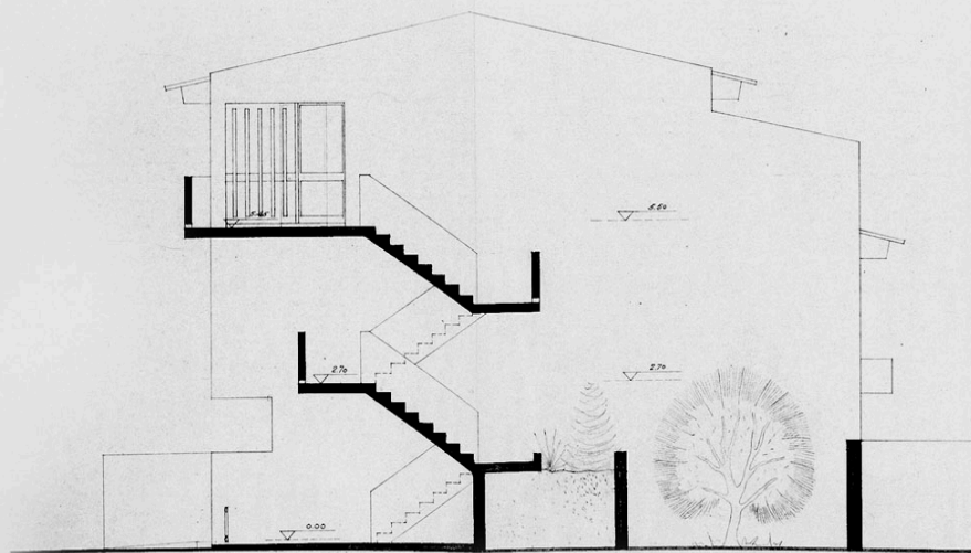
CORTE C-D
