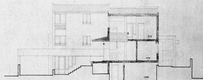
CORTE D-D
