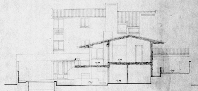
CORTE B-B
