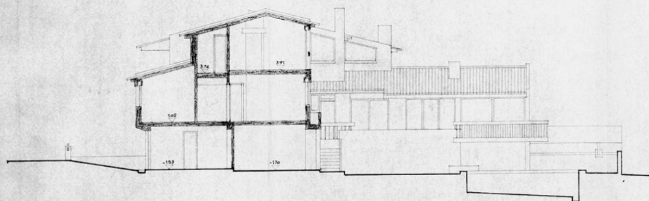
CORTE C-C
