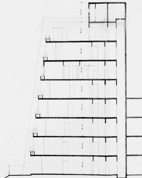
CORTE A-B
