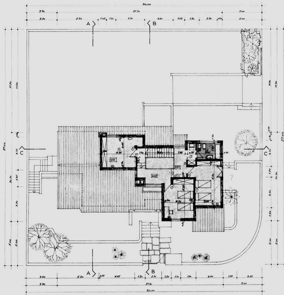
PLANTA DO 1º ANDAR
