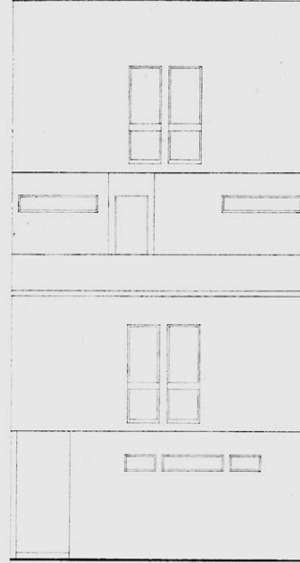
ALÇ. DE TARDOZ
