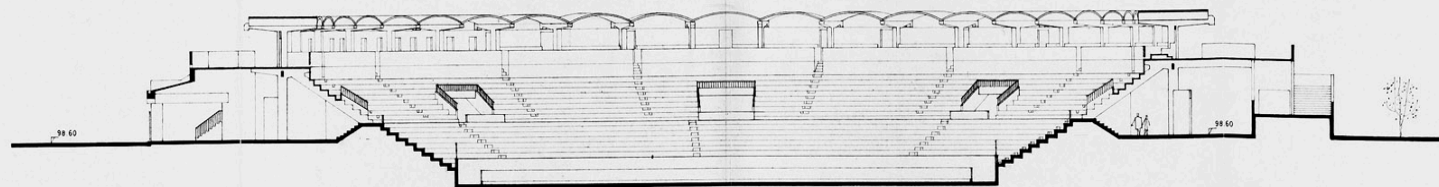
CORTE 1
