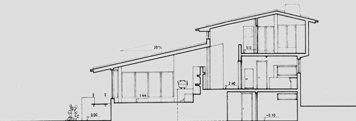
CORTE B-B
