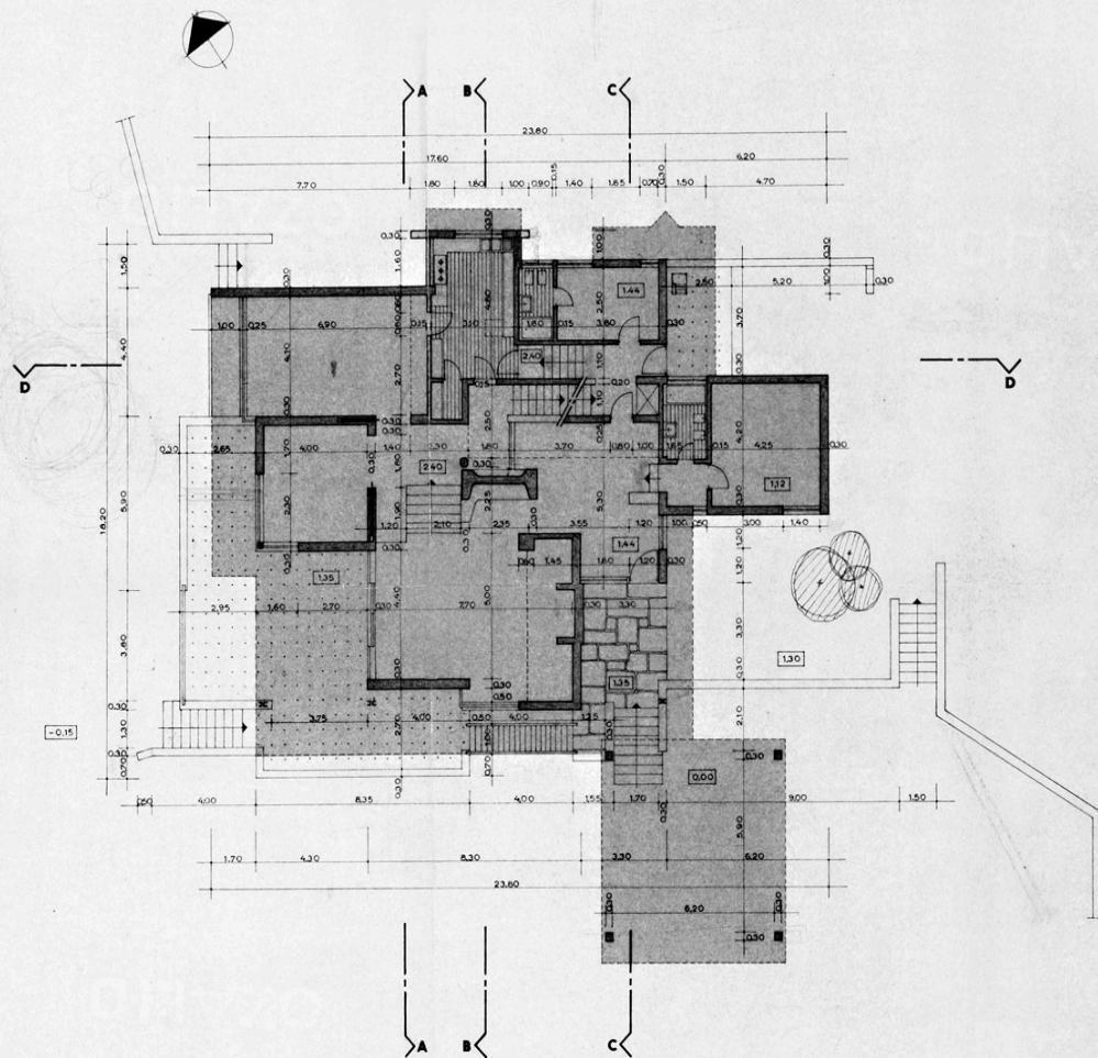
PLANTA DO RÊS DO CHÃO
