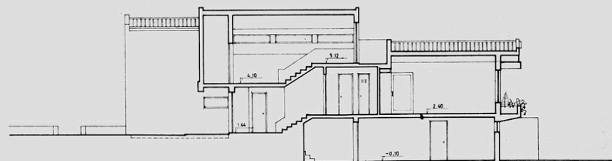
CORTE D-D
