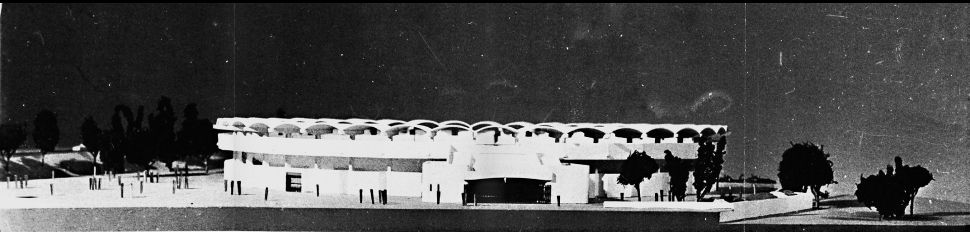
ALÇADO POENTE
