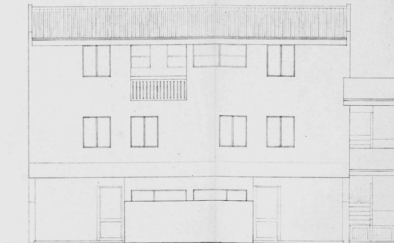
ALÇADO DA FRENTE
